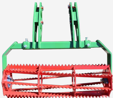
Réglage du rouleau par les axes goupillés. Rouleau barre de série adapté à la taille du cadre. Possibilité de demander d'autres types de rouleau et dimensions différentes
